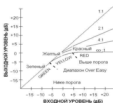
Рисунок 2: Кривая компрессии с перегибом OverEasy и светодиодные индикаторы THRESHOLD
